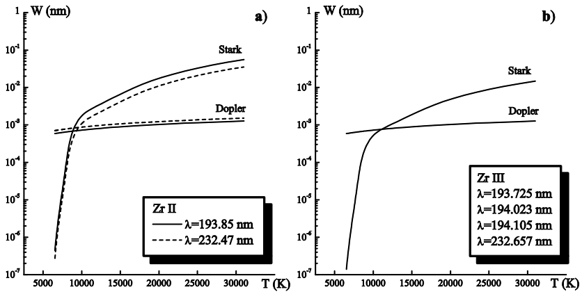
СЛИКА II. Понашање Штаркових и Доплерових ширина (FWHM) са температуром, за моделе звезданих атмосфера са T_{\text{eff}}=10500 \text{ K} , \log g=4.0 и V_1=0.08 \text{ km s}^{-1} за а) \text{Zr II } 4d5s5p^2D^{\circ}_{3/2} - 4d^25s a^2D_{3/2} , \lambda=193.85 \text{ nm} (пуна линија) и \text{Zr II } 4d5s5p y^2F^{\circ}_{5/2} - 4d^25s b^2G_{7/2} , \lambda=232.47 \text{ nm} (испрекидана линија), и б) \text{Zr III } 4d^2^3P_1 - 4d5p^3P_0 , \lambda=193.725 \text{ nm} , \text{Zr III } 4d^2^1G_4 - 4d5p^1F_3 , \lambda=194.023 \text{ nm} , \text{Zr III } 4d^2^3P_2 - 4d5p^3P_0 , \lambda=194.105 \text{ nm} и \text{Zr III } 4d^2^3P_1 - 4d5p^3P_0 , \lambda=194.657 \text{ nm} . На Сл. IIб није показана зависност од температуре за све наведене линије пошто је приближно једнака.
