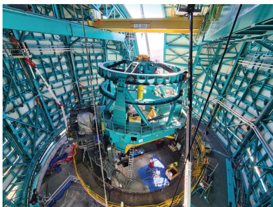
Слика 1. Лево: LSST 3.2-гигапикселна дигитална камера и Симонијев телескоп за преглед неба. Троделни систем огледала телескопа (8.4 m, 5 m и 3.4 m) омогућава брзо и прецизно усмеравање у року од приближно 5 секунди. Извор фотографије: Rubin Obs/NSF/AURA. Десно: Слика из Deep Lens Survey (DLS), која открива десет пута више галаксија по јединици површине у односу на Sloan Digital Sky Survey (SDSS), док ће LSST покривати 50.000 пута већу површину у шест оптичких филтера. Извор фотографије: Deep Lens Survey / UC Davis / NOAO.
