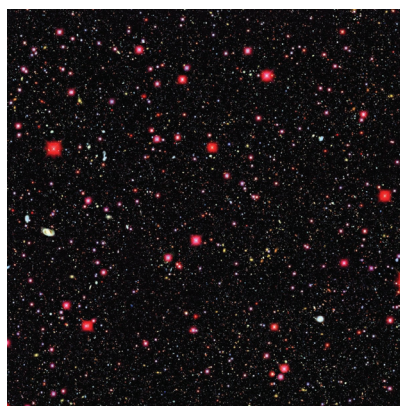
Слика 1. Лево: LSST 3.2-гигапикселна дигитална камера и Симонијев телескоп за преглед неба. Троделни систем огледала телескопа (8.4 m, 5 m и 3.4 m) омогућава брзо и прецизно усмеравање у року од приближно 5 секунди. Извор фотографије: Rubin Obs/NSF/AURA. Десно: Слика из Deep Lens Survey (DLS), која открива десет пута више галаксија по јединици површине у односу на Sloan Digital Sky Survey (SDSS), док ће LSST покривати 50.000 пута већу површину у шест оптичких филтера. Извор фотографије: Deep Lens Survey / UC Davis / NOAO.
