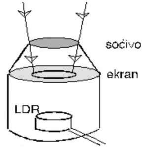
Слика 6: Сочиво, мутни екран, и фотоотпорник, чине једноставан и веома осетљив фотометар.
