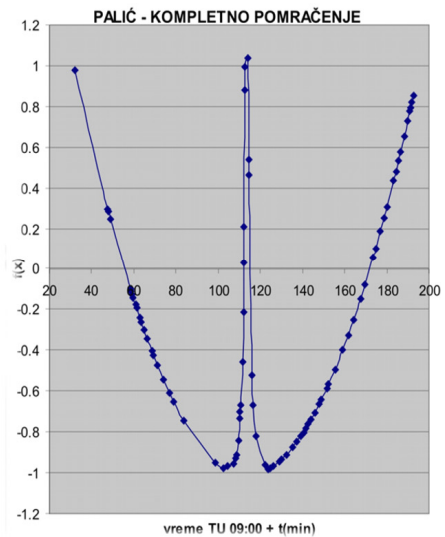
Слика 7: Теоријски модел који обухвата све три врсте помрачења (лево) и криве добијене из посматрања помрачења 11. августа 1999. на Палићу (десно).
