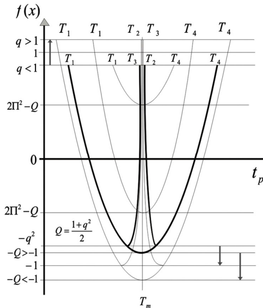
Слика 7: Теоријски модел који обухвата све три врсте помрачења (лево) и криве добијене из посматрања помрачења 11. августа 1999. на Палићу (десно).
