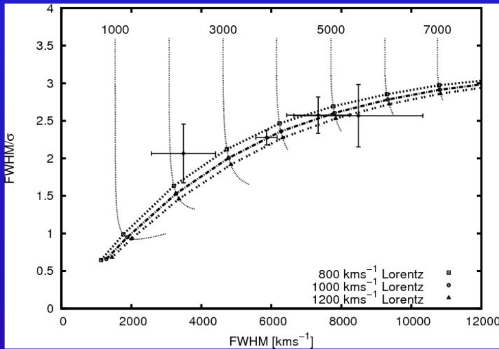
HeII \lambda 4686
