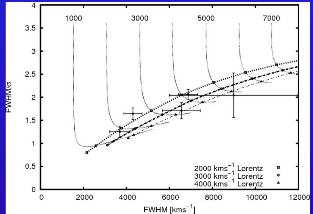
CIV \lambda 1550
